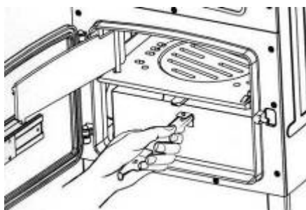
Bild 6 – Aschekasten
