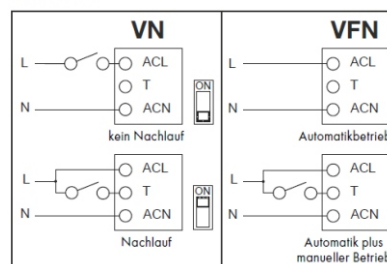
Schaltbild
