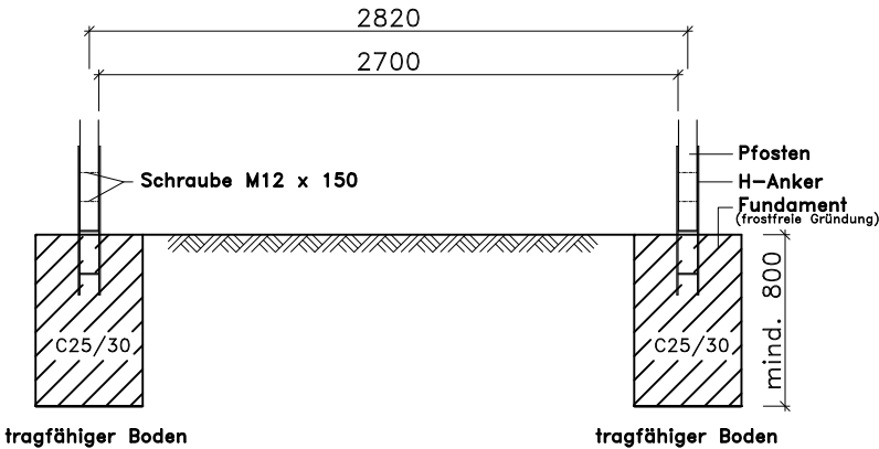
Schnitt B-B
