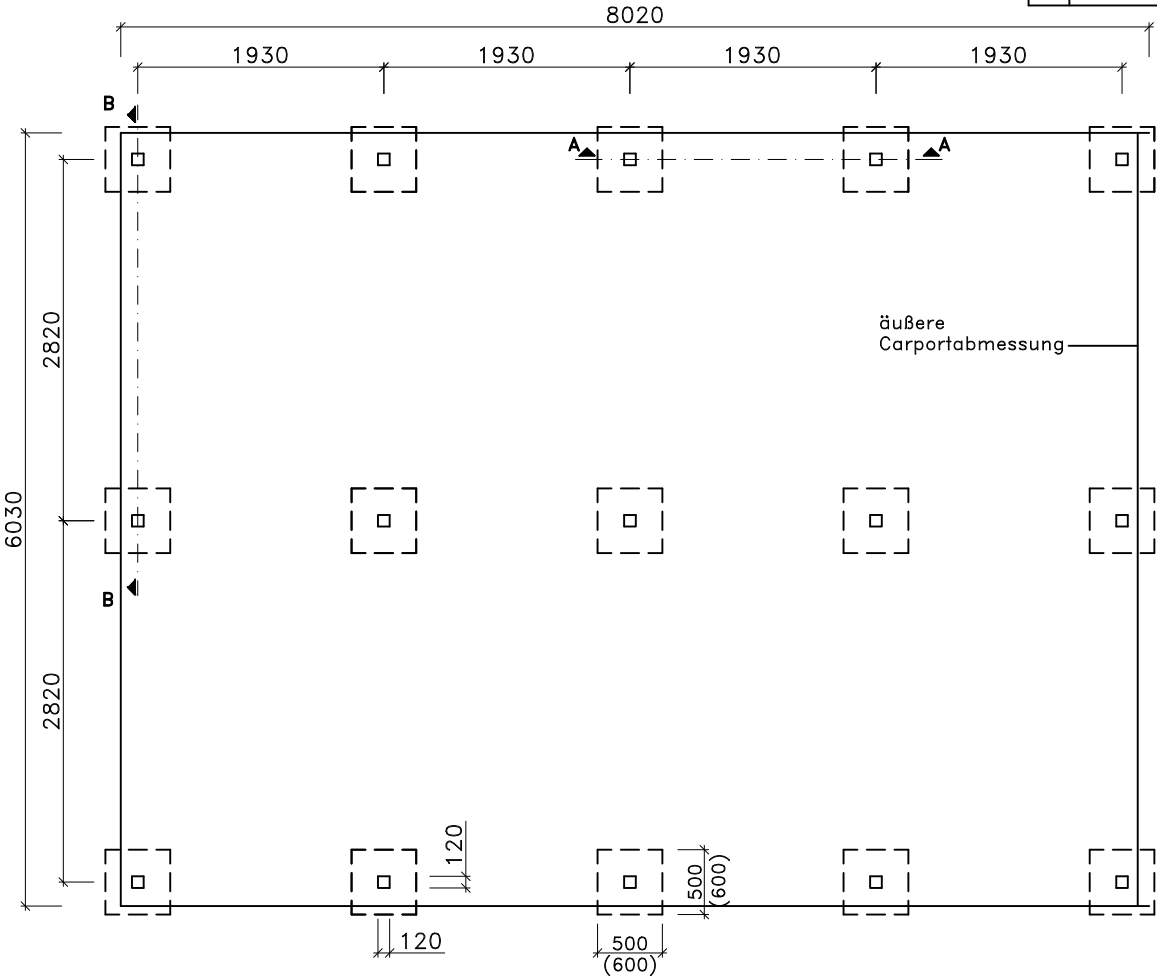
Grundriß
